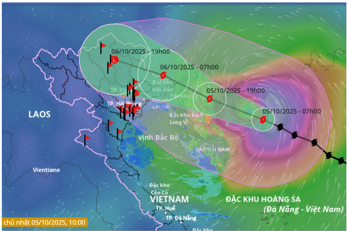
Vị trí và hướng đi của bão số 11
