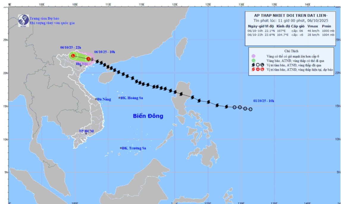
Đường đi của áp thấp nhiệt đới trưa 6/10
