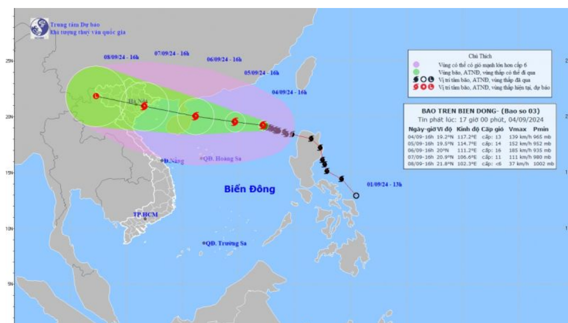
Vị trí và đường đi của bão số 3
