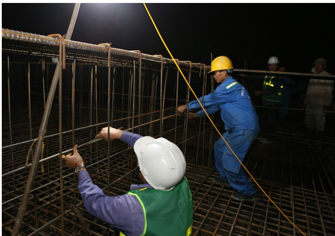
Thi công móng xuyên đêm vị trí 288 đường dây 500kV NMNĐ Nam Định 1 - Phố Nối - Ảnh:VGP/Toàn Thắng
