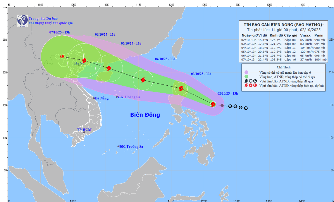
Hướng di chuyển của bão Matmo. Ảnh: KTTV
