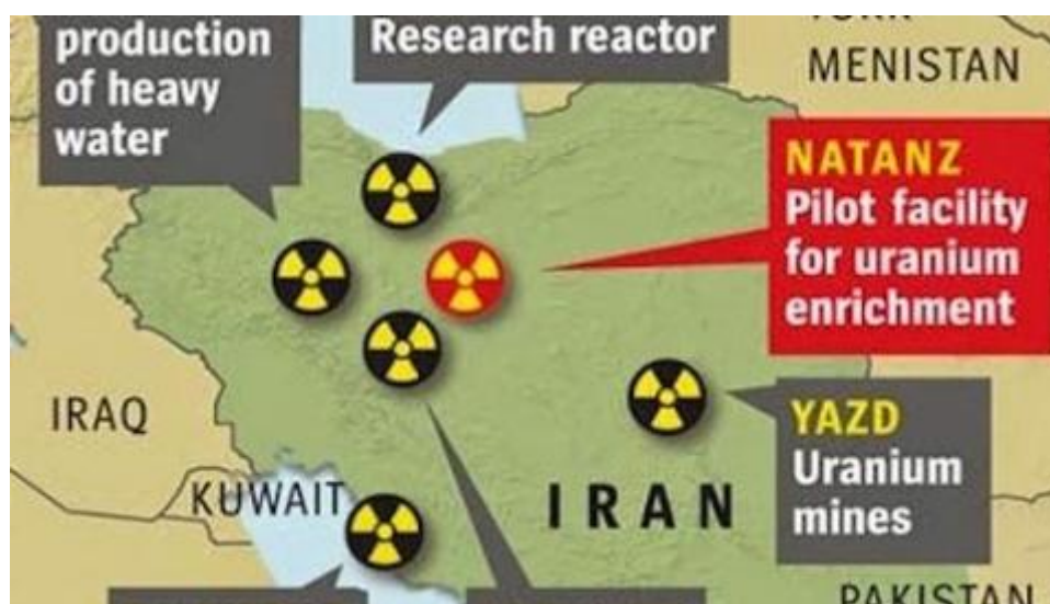
Bản đồ các cơ sở hạt nhân chủ chốt (đã biết) trên lãnh thổ Iran
