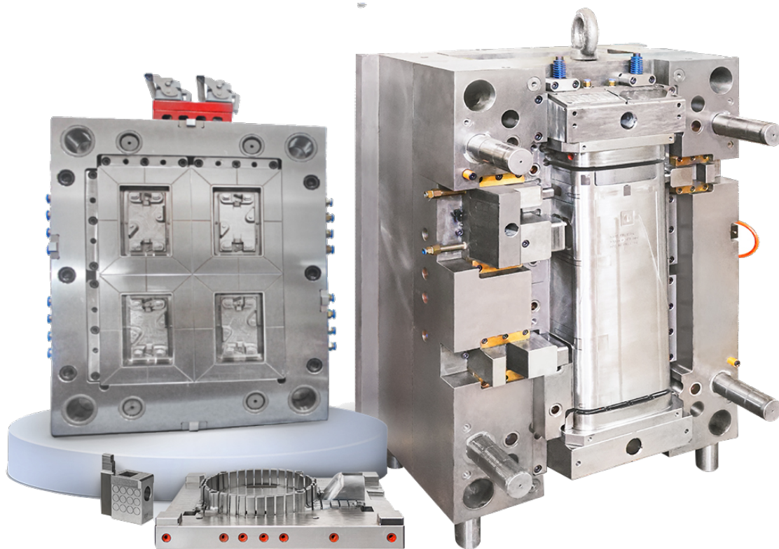
Khuôn mẫu bằng kim loại MIDA dùng trong công nghệ ép phun để tạo ra sản phẩm nhựa
