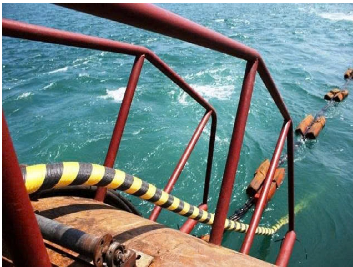
Những mét cáp điện ngầm 22kV được đơn vị thi công rải xuống biển trên đoạn Ba Mùn - Cô Tô
