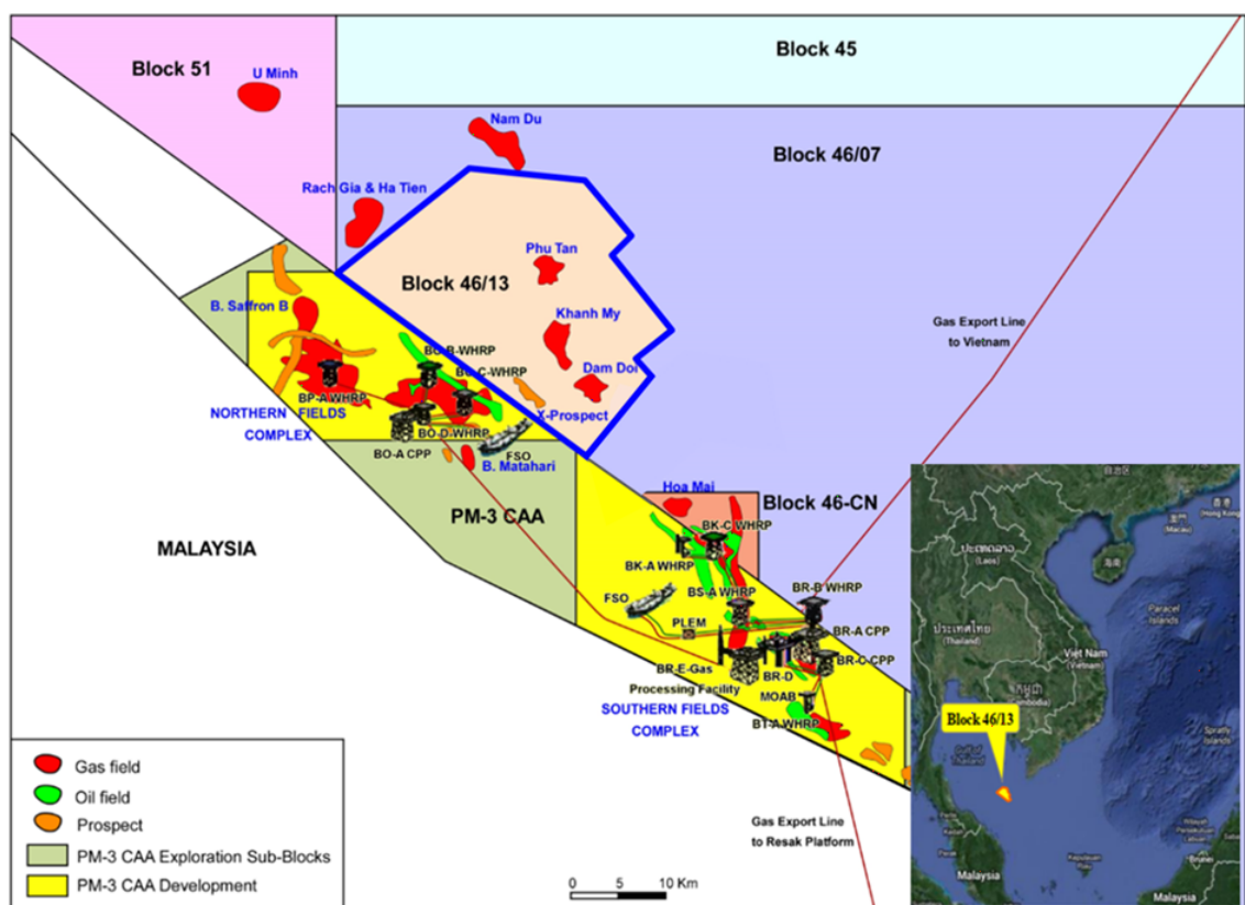
Sơ đồ phát triển mỏ Khánh Mỹ - Đầm Dơi (Lô 46/13) và Lô PM3 CAA
