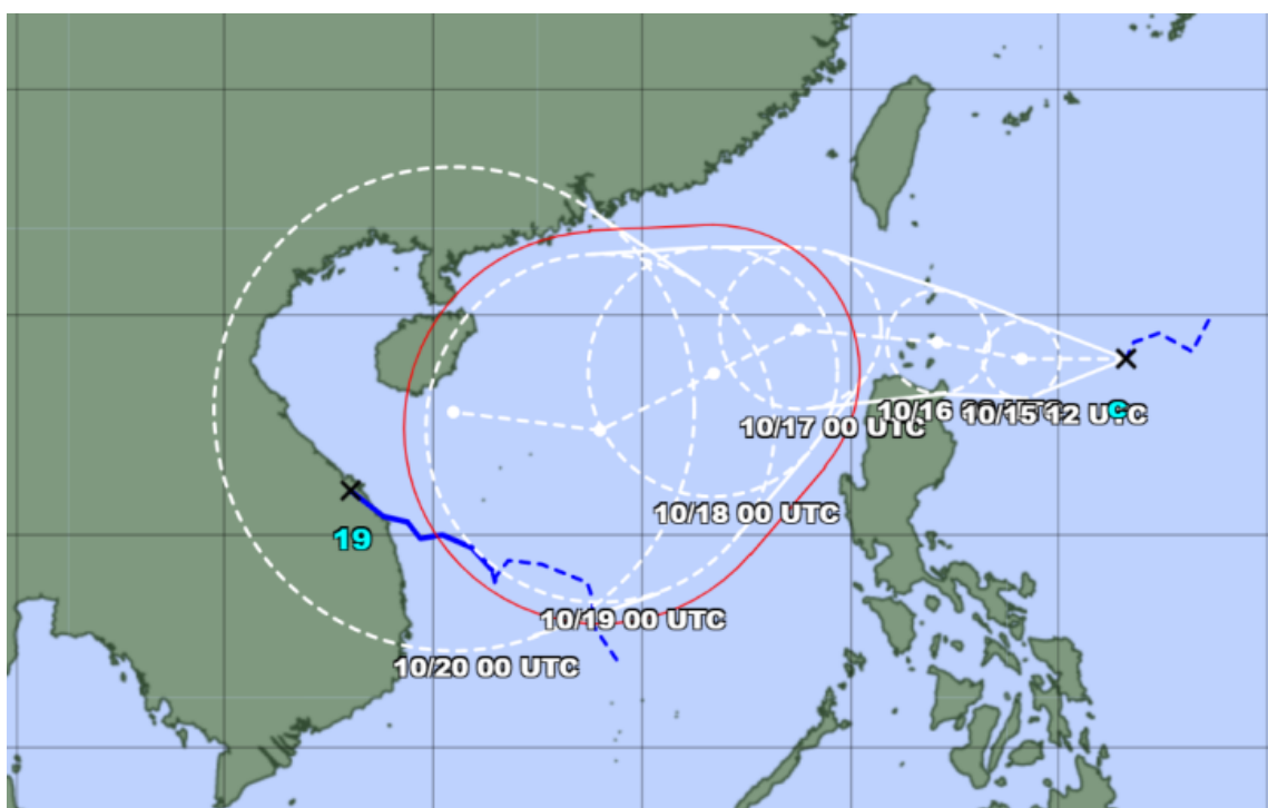
Dự báo đường đi cơn bão của cơ quan khí tượng Nhật Bản..
