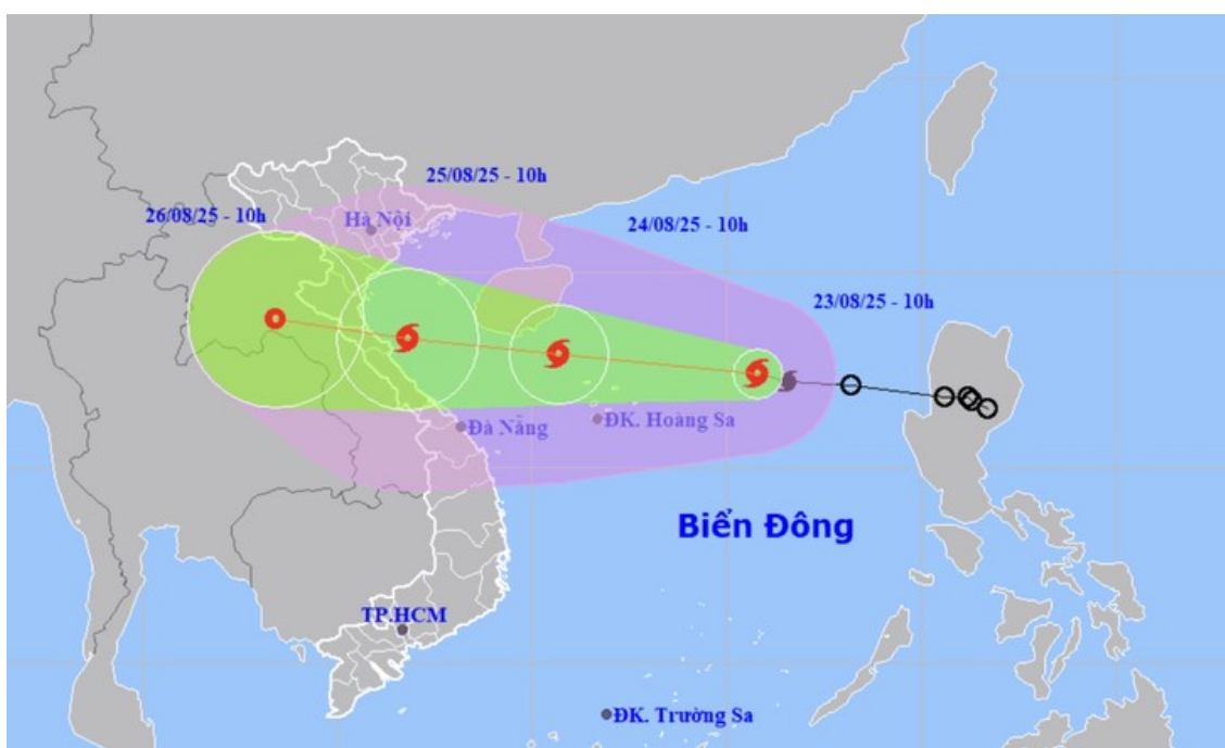
Dự báo vị trí và hướng di chuyển bão số 5 lúc 10h sáng 23/8 - Ảnh: NCHMF
