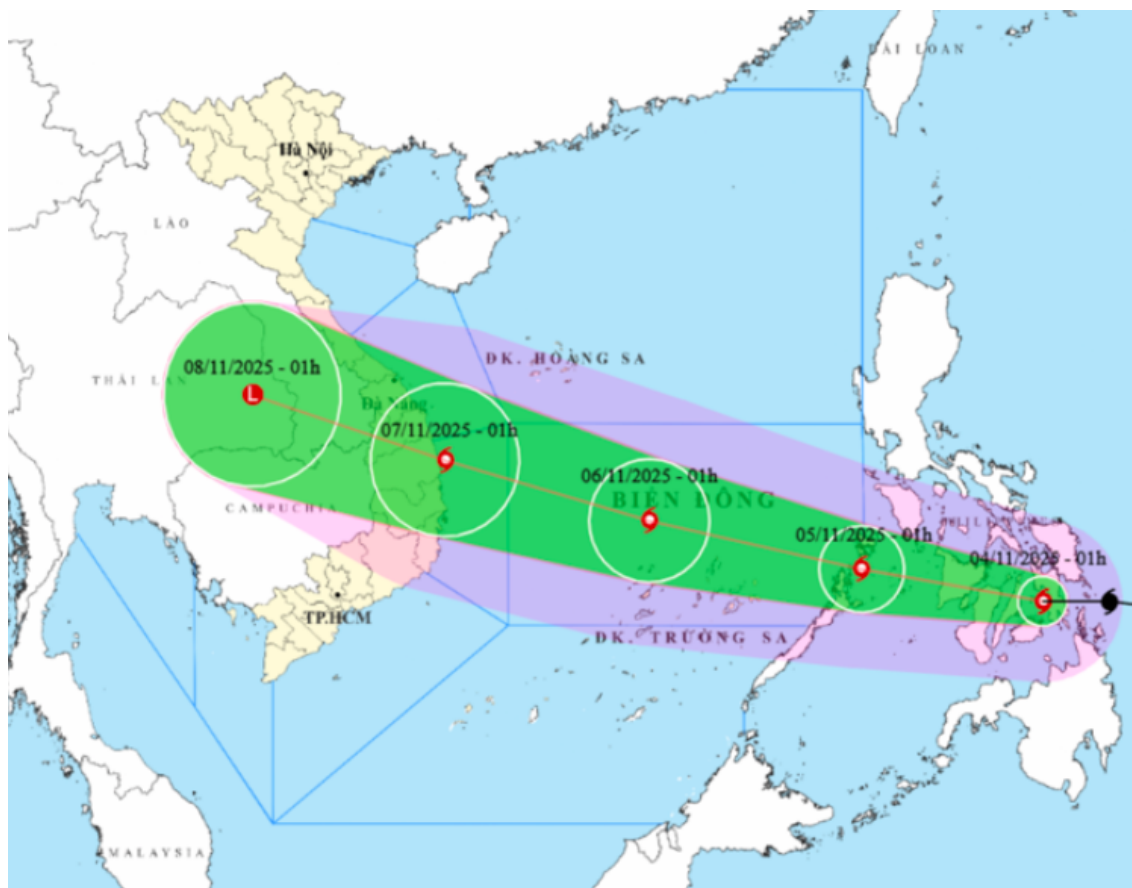
Hướng di chuyển của bão Kalmaegi lúc 1 giờ ngày 4/11 (Ảnh: Trung tâm Dự báo khí tượng thủy văn quốc gia)
